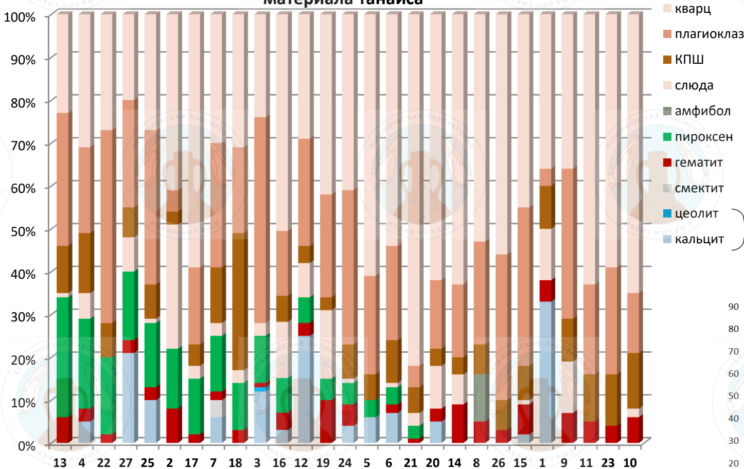
Минеральный состав кристаллической фазы краснолакового материала Танаиса
